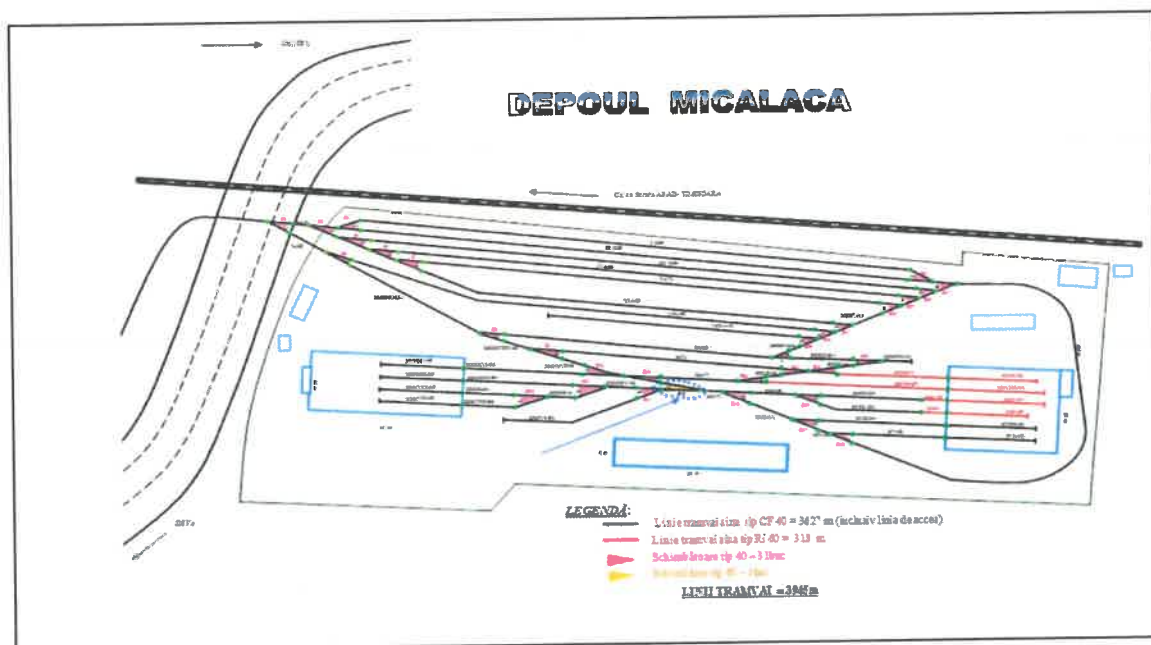
Planul general al depoului Micălaca
